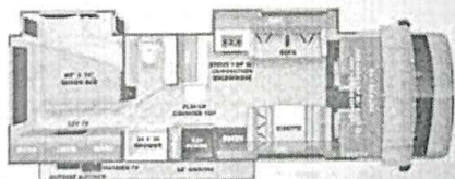
2860DS (Available on Ford E450)
